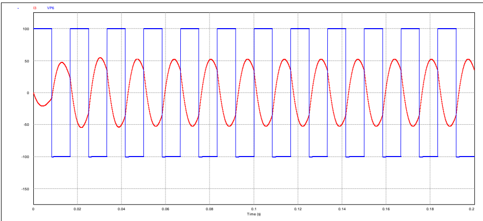
Rys. 4. Przebiegi napięcia i prądu odbiornika RLC
